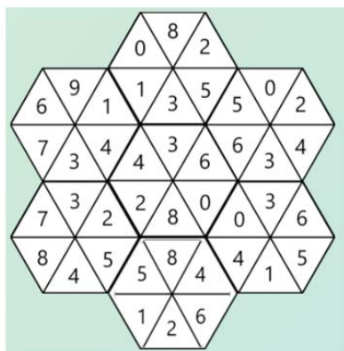
2. Ábra – A hexagonos játék helyes megoldása
