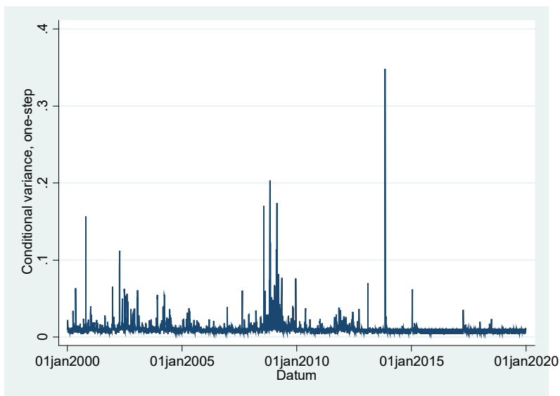
3. ábra: A korona euróval szembeni napenkénti volatilitása 2000.01.01. – 2019.12.31. között
